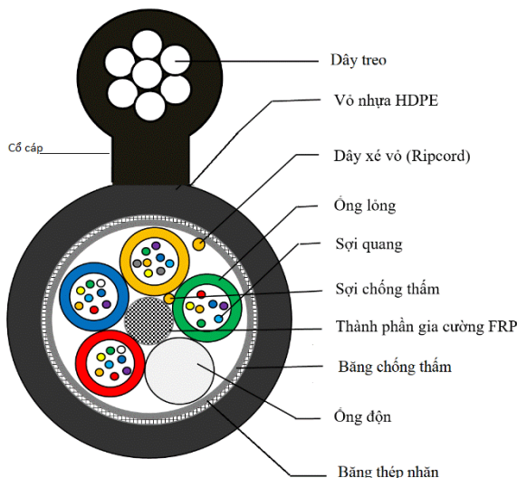
Bảng 1 - Cấu trúc và các thành phần của cáp sợi quang treo hình số 8 có vỏ bọc kim loại
